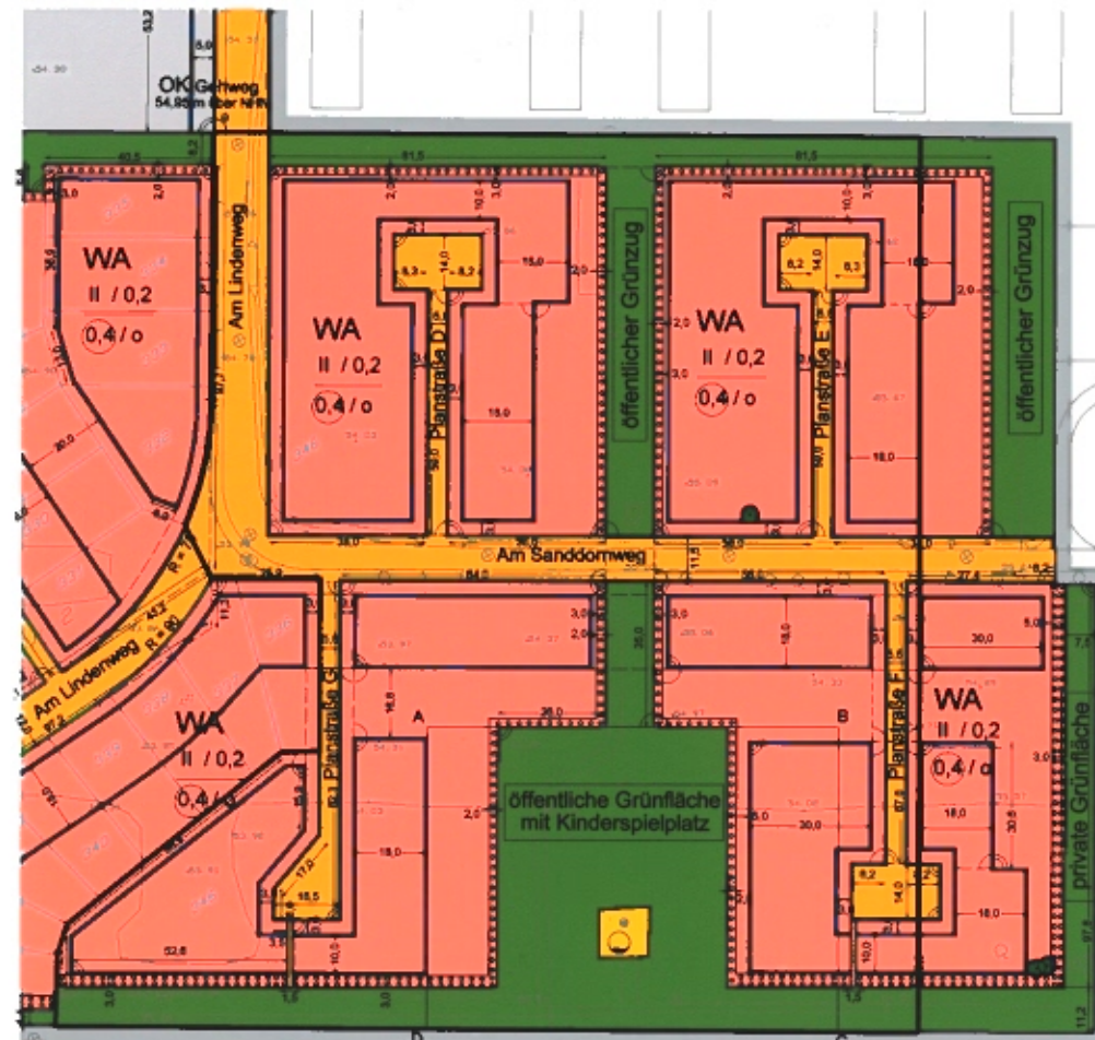
Ausschnitt B-Plan Lindenring M 1: 2000
